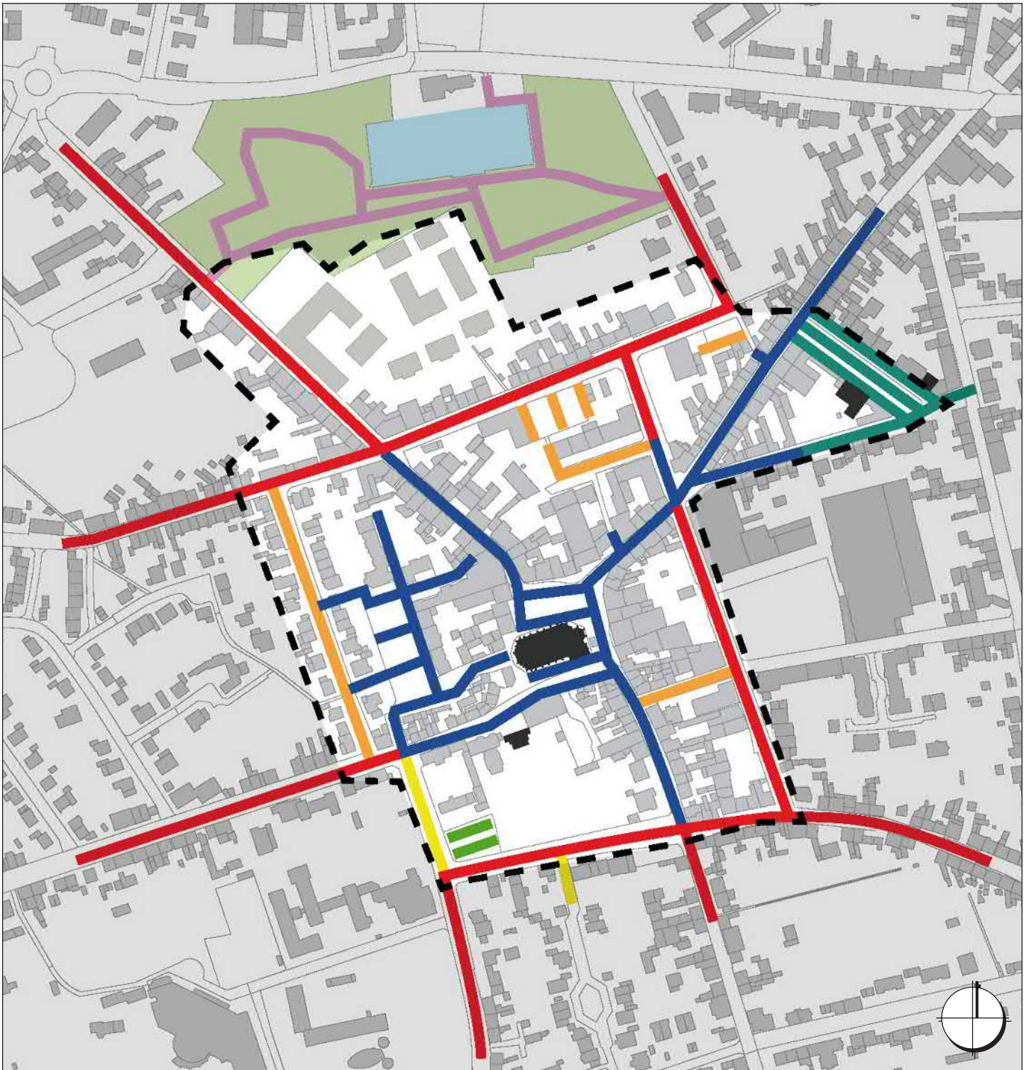
Lageplan 03: Leuchtenbestand
