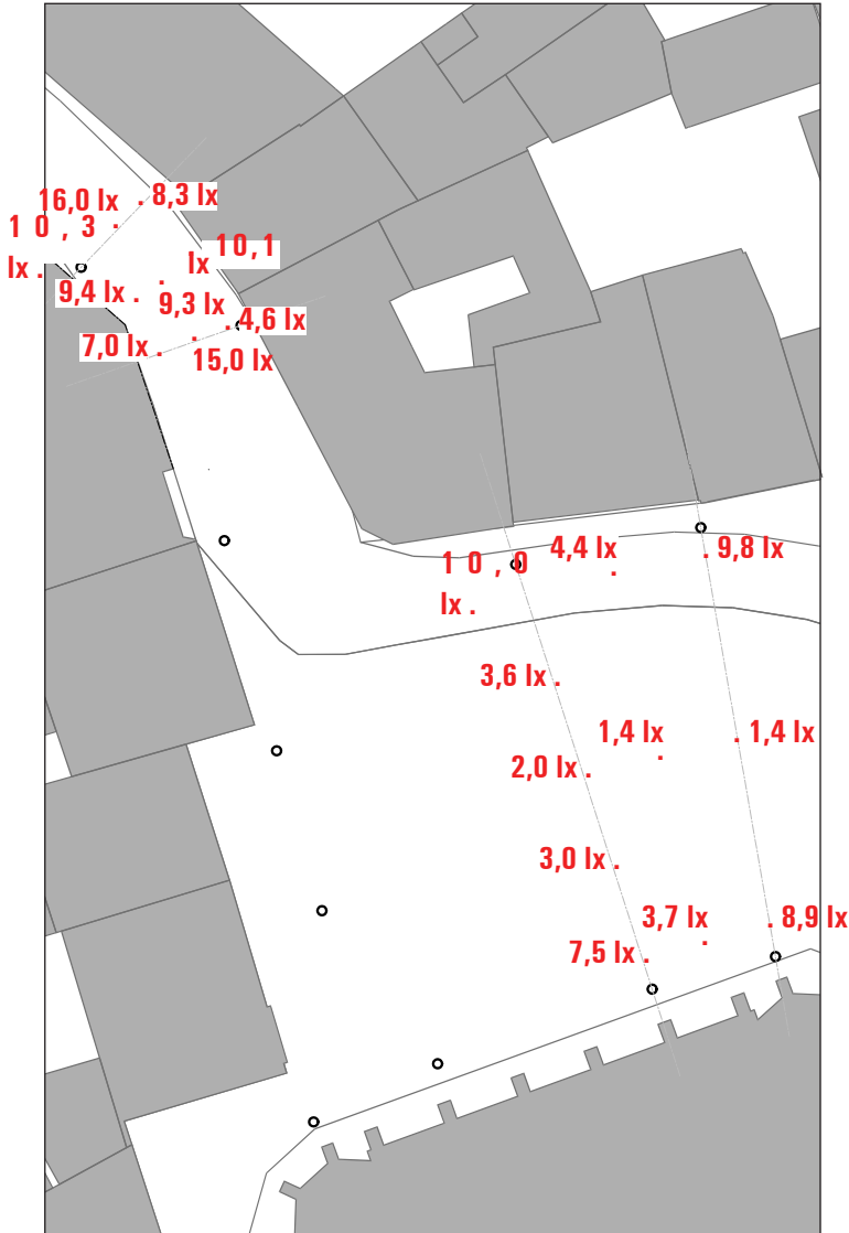
Lichtmessung Marktplatz und Bahnstraße mit historisierenden Altstadtleuchten
