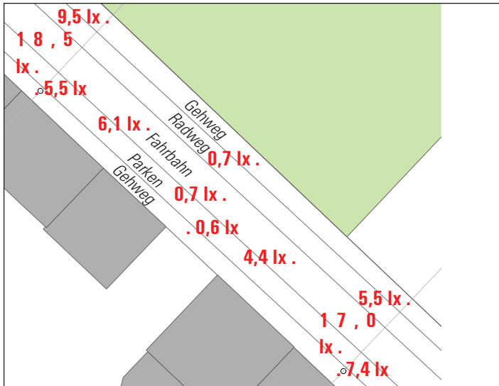
Lichtmessung Bahnstraße mit Mastaufsatzleuchten
