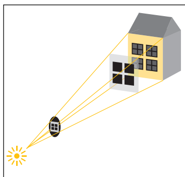
Funktionsprinzip Gobo-Maske
