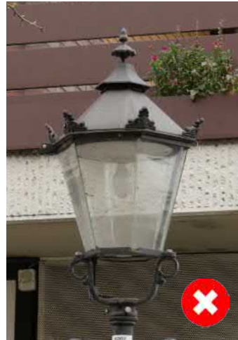
Freistrahkende NAV-Lichtquelle ohne Lichtlenkung in historisierender Mastleuchte
