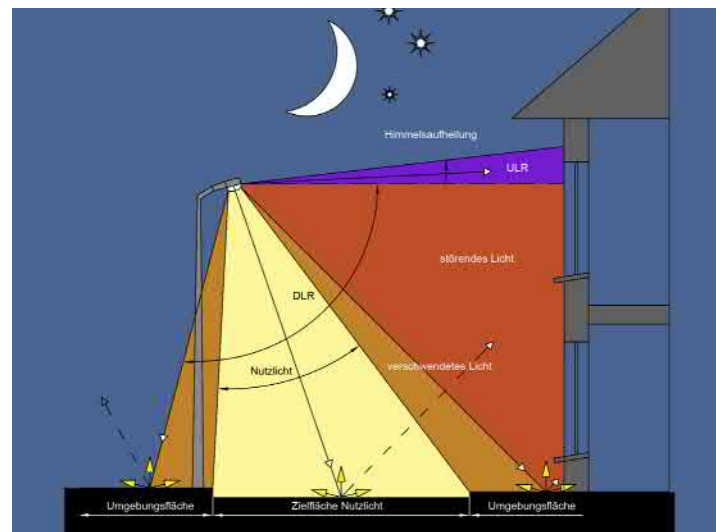
Strahlungszonen von Außenleuchten / Quelle: Irs
