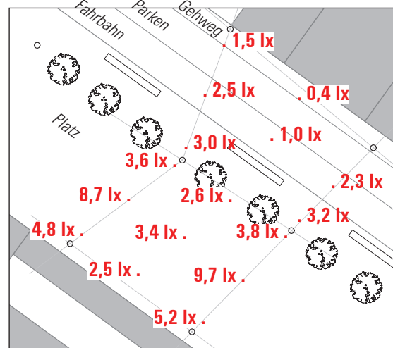
Lichtmessung Kaiserplatz mit Sonderleuchten
