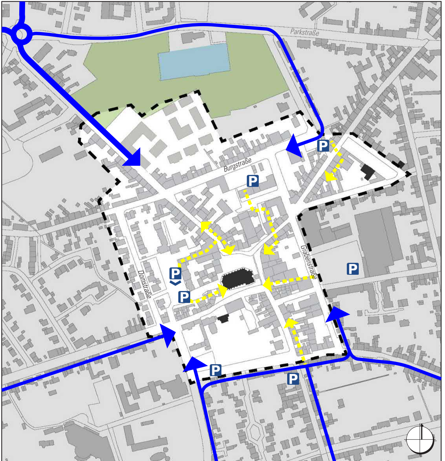
Lageplan 04: Stadteingangssituationen
